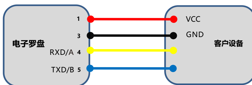
UART,RS232/RS485 接线图
