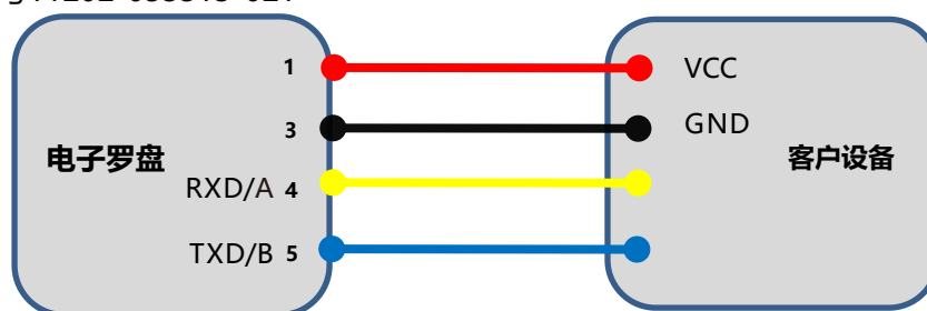
UART,RS232/RS485 接线图
