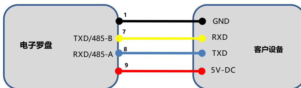
UART,RS232/RS485 接线图
